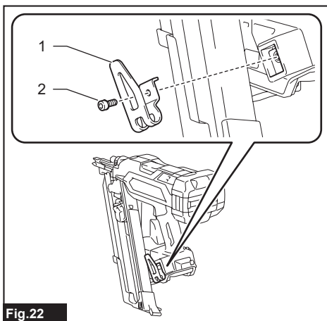
► 1. Gancho en forma de clip 2. Perno hexagonal
