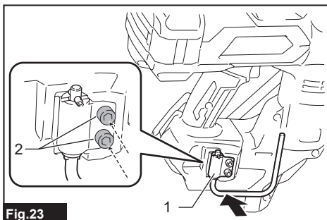
► 1. Gancho en forma de C 2. Pernos hexagonales
